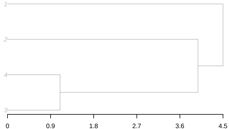
Parasite Phylogeny
